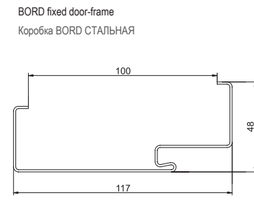
BORD corner steel door-frame Коробка BORD СТАЛЬНАЯ угловая
