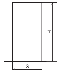
Dimensions of holes in the wall for fixed door frame assembly Размеры дверного проема для установки фиксированной дверной коробки
