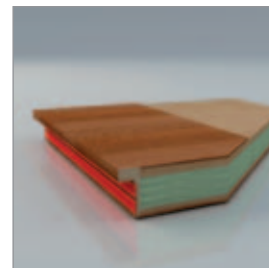
Strengthened fire resistant construction of the fire door leaves. Укрепленная огнеустойчивая конструкция противопожарных дверей
