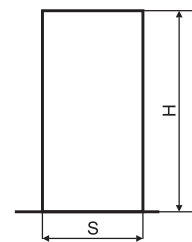
Dimensions of holes in the wall for Standard 2-pack door frame assembly Размеры дверного проема для установки коробки Standard 2-pack
